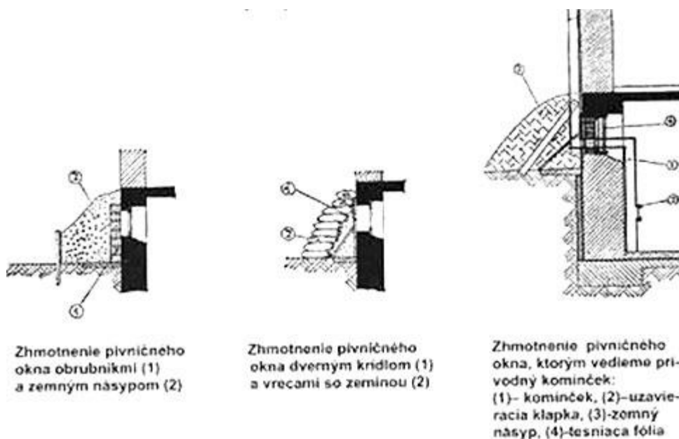
Obr. Grafické znázornenie úprav okien pri budovaní jednoduchých úkrytov
